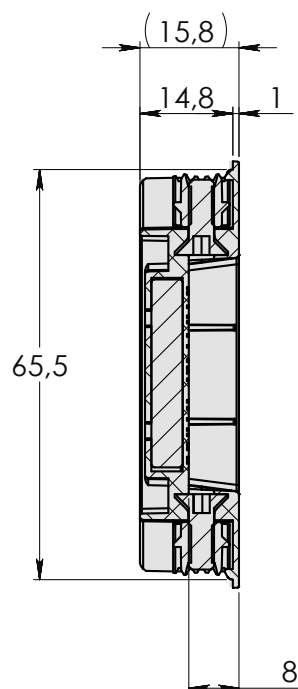
SEZIONE B-B SCALA 1 : 1
