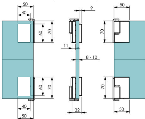
HINGE DIMENSIONS
