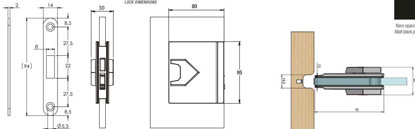
DIMENSIONI SERRATURA LOCK DIMENSIONS
